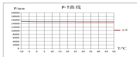
功率温度变化曲线
